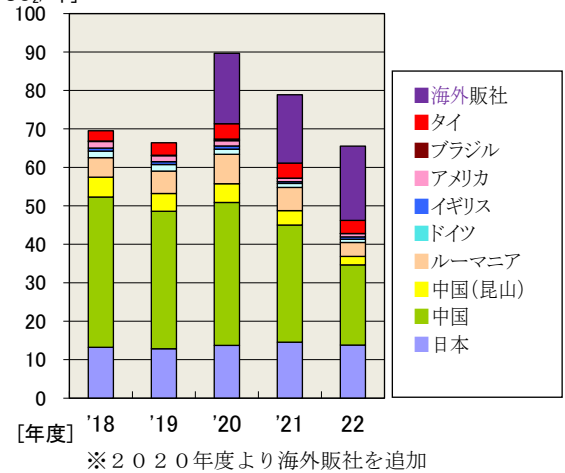
[千 t-CO 2 /年] グローバル GHG 排出量
