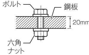
普通ボルト
