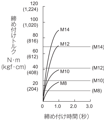
普通ボルト
