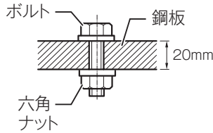
普通ボルト
