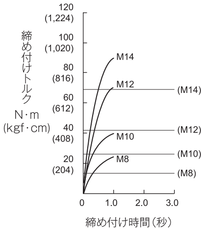
普通ボルト
