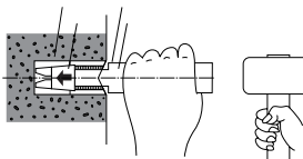
プラグプラグ内装アンカ用打込棒
