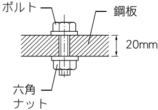
普通ボルト
