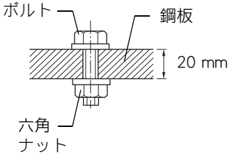
普通ボルト
