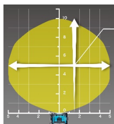
ML809の照射範囲 (照度70lx以上の範囲)
