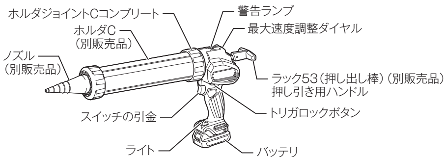
ホルダC (800mL)仕様 (ホルダC (800mL)は別販売品になります。)
