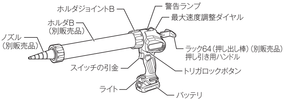
ホルダB (600mL)仕様 (ホルダB (600mL)は別販売品になります。)
