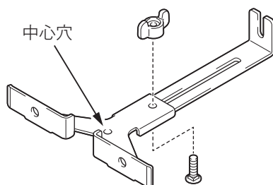
〔半径121 ～ 221 mm の円を加工する場合〕
