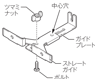
〔半径70 ～ 121 mm の円を加工する場合〕
