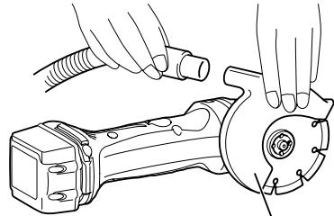
集じんアタッチメント
