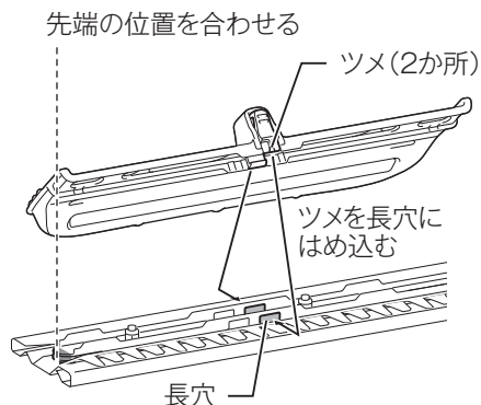
標準刃
