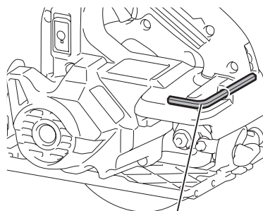
六角棒スパナ5 [イラストはHS475D]
