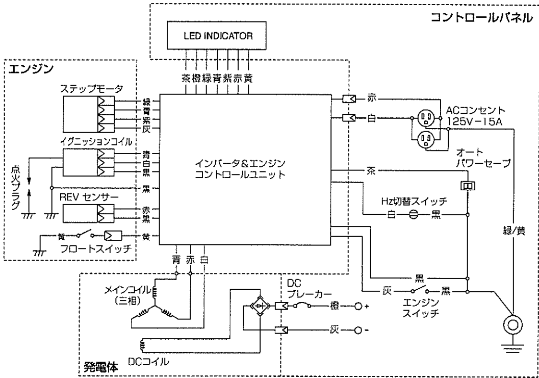
結線図
