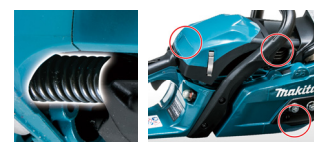
金属スプリング(左)とその採用箇所
