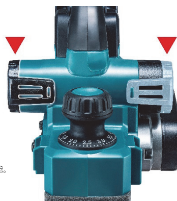
切削屑両側排出 ダクトを付替える事で排出方向を変更可能。
